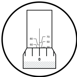
Bild 3: Beispieleinstellung 50 Nm
