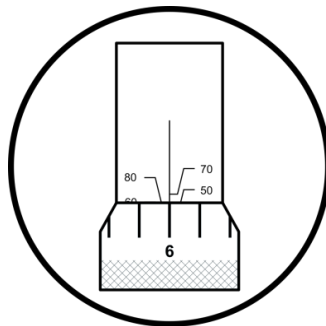
Bild 4: Beispieleinstellung 56 Nm
