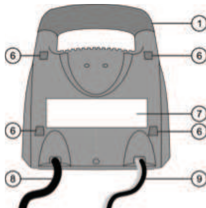
Illustration 2 : Vue arrière
