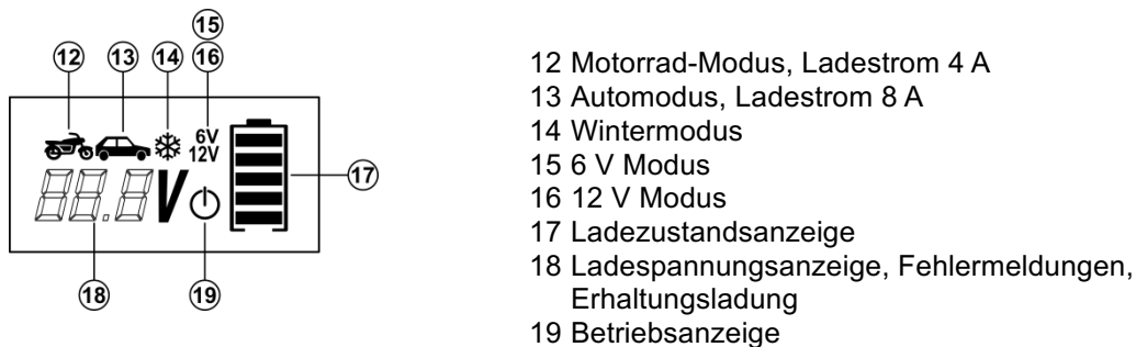
Bild 3: Display
