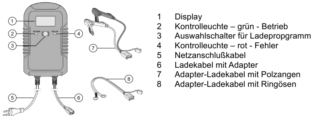
Bild 1: Ansicht Vorderseite
