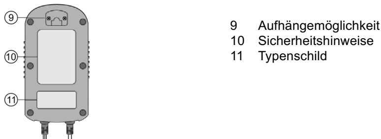
Bild 2: Ansicht Rückseite
