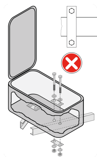
Montage op een V-dissel
