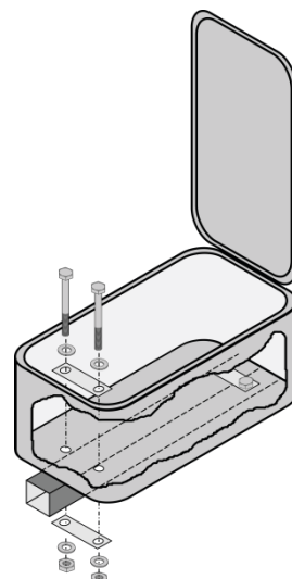
Montage auf einem Vierkant-Zugrohr quer / längs
