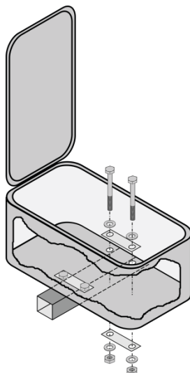
Montage sur un tube de traction côté / longueur
