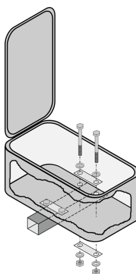
Montage op een vierkante trekstang dwars/overlangs
