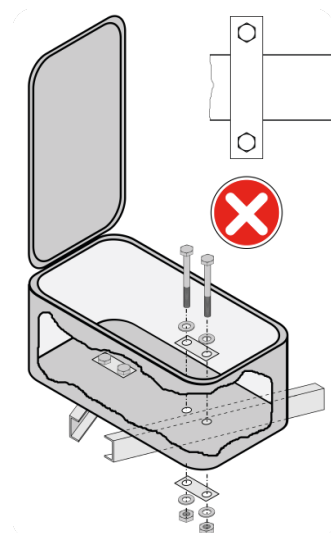
Montage auf einer V-Deichsel
