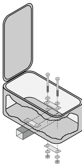
Prečna/vzdolžna montaža na oglati vlečno cev
