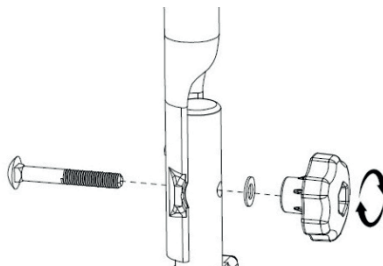
Bild 3: Festschrauben U-Bügel
