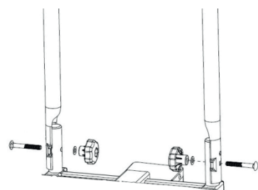
Figura 2: Montaggio staffa a U
