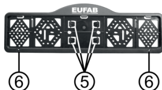
Figura 6: Montaggio targa
