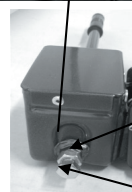
Vis de réglage pour la fermeture rapide
