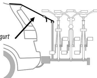
Bild 21: Zugentlastungsgurt
