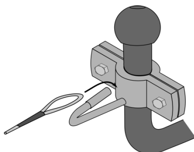
Bild 4: Einhängen des Abreißseils
