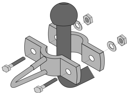
Afbeelding 1: Losse onderdelen
