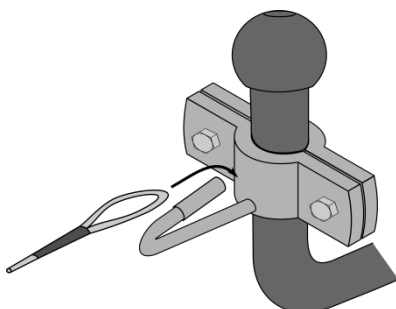
Afbeelding 4: De losbreekkabel inhangen
