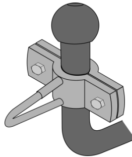
Bild 2: Halter am Kupplungshals montiert.
