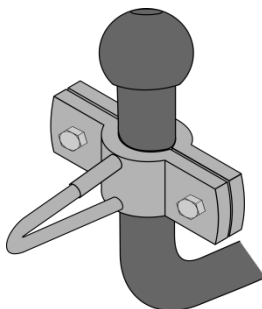
Afbeelding 2: Houder aan de koppelingshals gemonteerd.
