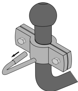
Afbeelding 3: De veerhuls terugtrekken
