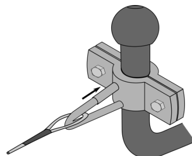
Afbeelding 5: De veerhuls sluiten
