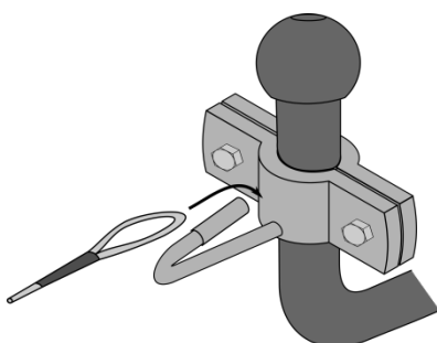
Figure 4 : Accrochage du câble de rupture d'attelage
