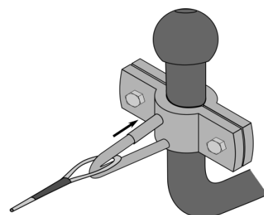
Bild 5: Schließen der Federhülse
