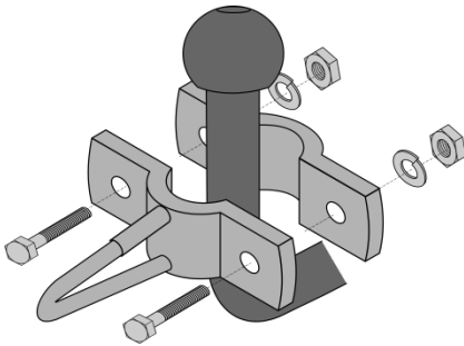
Bild 1: Einzelteile
