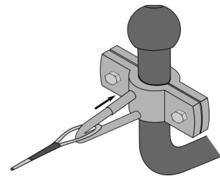
Bild 5: Schließen der Federhülse
